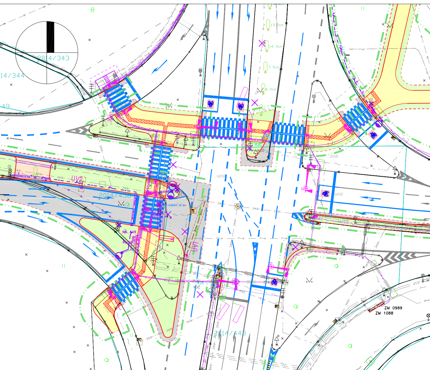
VÝŘEZ VNITŘNÍ KŘÍŽOVATKY BEZ POPISŮ 1:500
